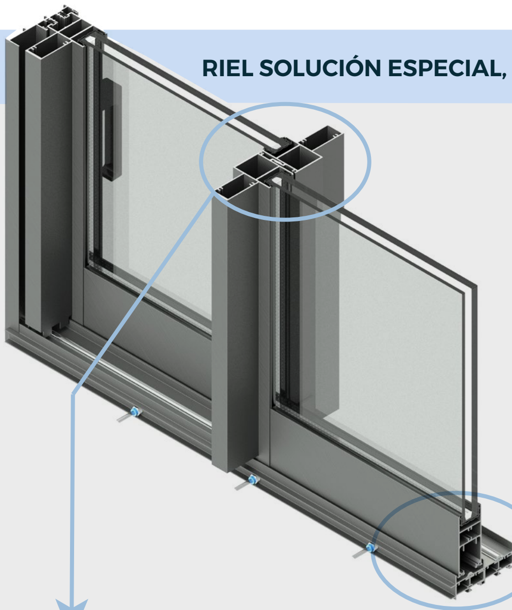
TRASLAPE REFORZADO
