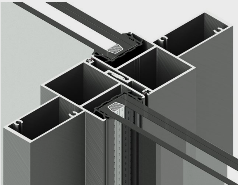
TRASLAPE REFORZADO
